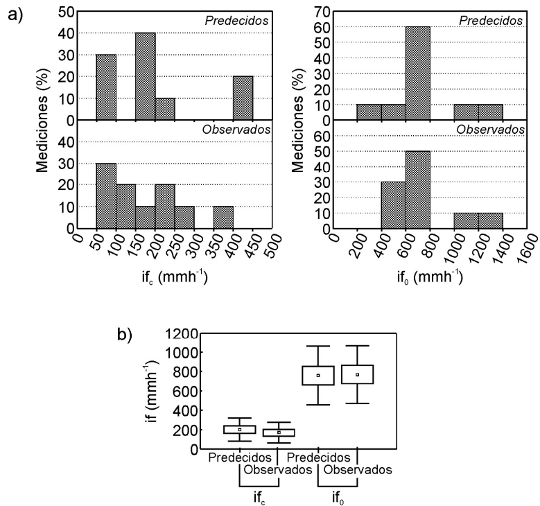
Figura 4. Condiciones de la calibración del modelo de Horton para las diferentes curvas de infiltración y sus valores de las tasas de infiltración inicial ( if_0 ) y final constante ( if_c ). a) Comparación de la distribución de los valores de if_0 e if_c observados y predecidos. b) Comparación de la variabilidad de if_0 e if_c registrada en los datos reales y en las curvas de Horton (la línea indica la desviación standard y los rectángulos el error standard).
