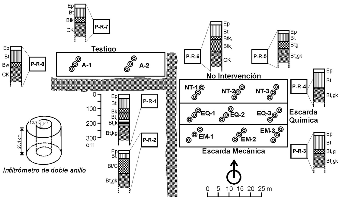
Figura 1. Esquema de situación de los ensayos de infiltración realizados sobre las parcelas experimentales y ubicación de los perfiles del suelo levantados en las lindes. A la izquierda se definen las dimensiones y morfología del infiltrómetro de doble cilindro usado en los ensayos.
