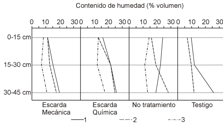
Figura 7. Variación del contenido de humedad antes de los ensayos en los diferentes tratamientos según los valores medios para los tramos 0-15 cm, 15-30 cm y 30-45 cm.
