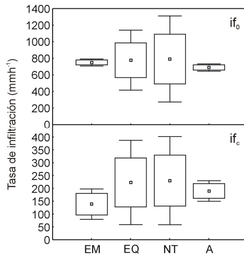
Figura 5. Gráfico Box & Wisher para comparar los valores de las tasas de infiltración inicial ( if_0 ) y final constante ( if_c ) en cada uno de los tratamientos. La línea indica la desviación standard y los rectángulos el error standard.
