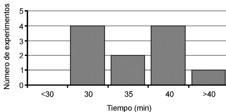
Figura 2. Frecuencia de duración de los ensayos de infiltración, mostrando el tiempo requerido hasta las condiciones de estabilización del volumen infiltrado.
