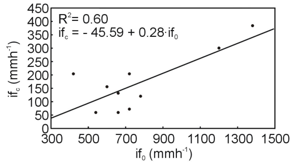
Figura 6. Relación entre tasa de infiltración final constante ( if_c ) e inicial ( if_0 ). Datos de todos los ensayos. Significativo estadísticamente para p < 0.05 .
