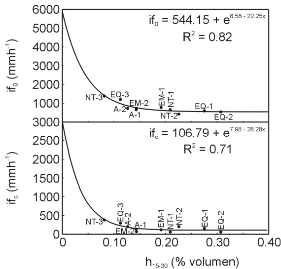
Figura 8. Relaciones entre las tasas de infiltración inicial ( if_0 ) y final constante ( if_c ) y el contenido medio de humedad a la profundidad de 15-30 cm. Ambas son significativas estadísticamente para p < 0.05 .
