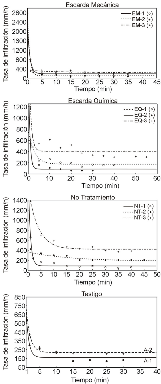
Figura 3. Curvas de infiltración para los diferentes ensayos según el modelo de Horton. El ensayo en EM-3 no permitió convergencia, pero se muestra una curva teórica para aproximar el proceso.
